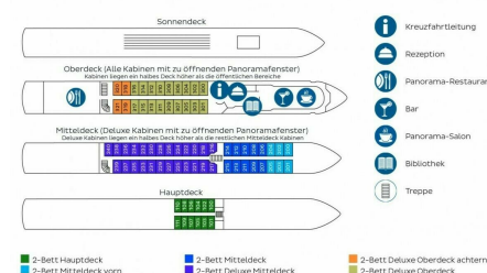
Deckplan MS BIJOU DU RHÔNE
